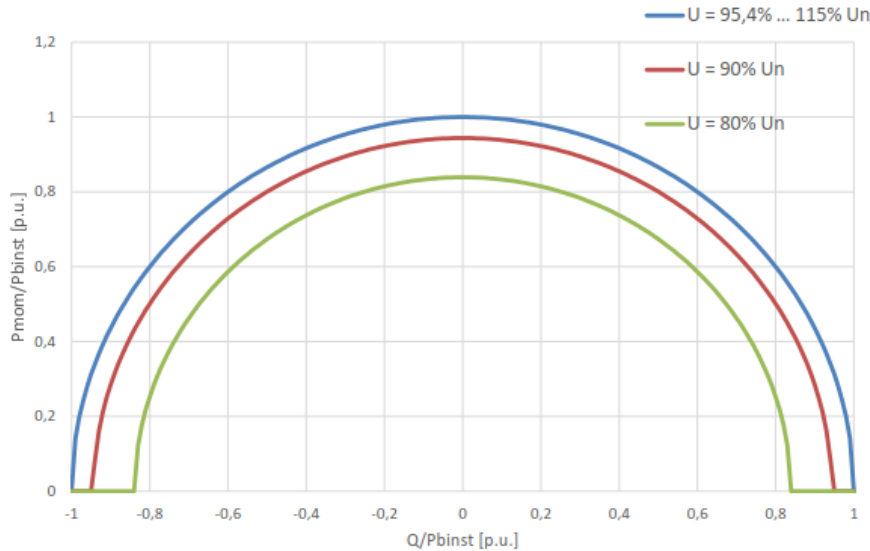
Abbildung 2 – P/Q -Diagramm gemäß Herstellererklärung
