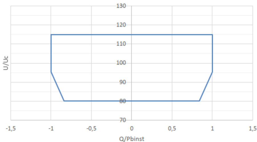
Abbildung 3 – Q(U) -Diagramm gemäß Herstellererklärung
