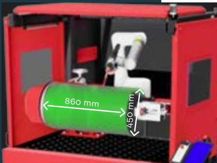
Bauteildimensionen mit Dreheinheit
